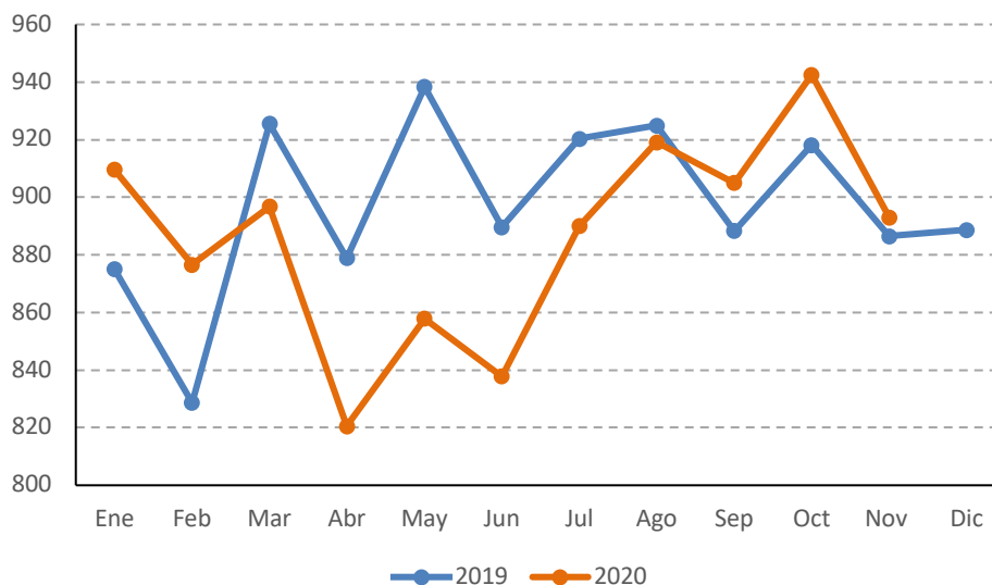
Gráfico 25. Demanda de electricidad, 2019-2020 GWh
