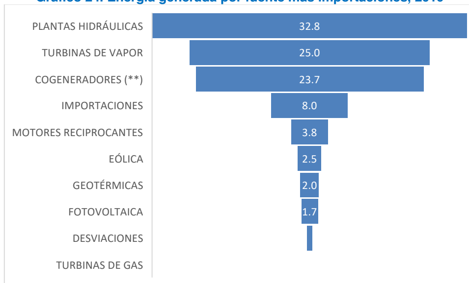
Gráfico 24. Energía generada por fuente más importaciones, 2019
