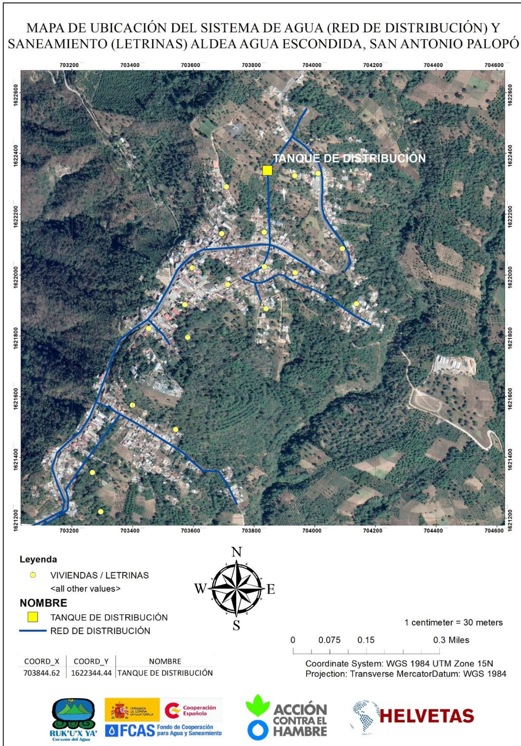
Ilustración 1: Mapa de ubicación del sistema de agua (red de distribución) y saneamiento, Aldea Agua Escondida
