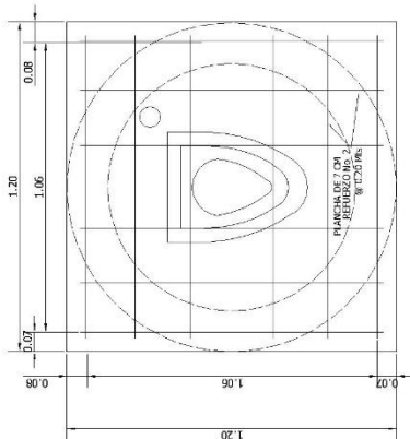
PLANTA BASE DE CONCRETO ESCALA 1/10
