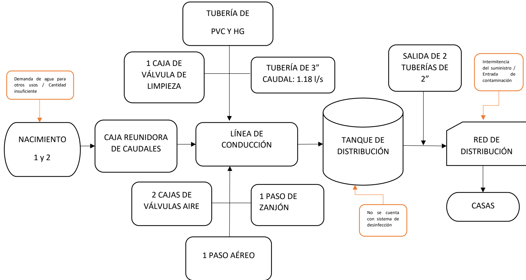
Ilustración 2: Diagrama de flujo del proceso del sistema de agua evaluado
