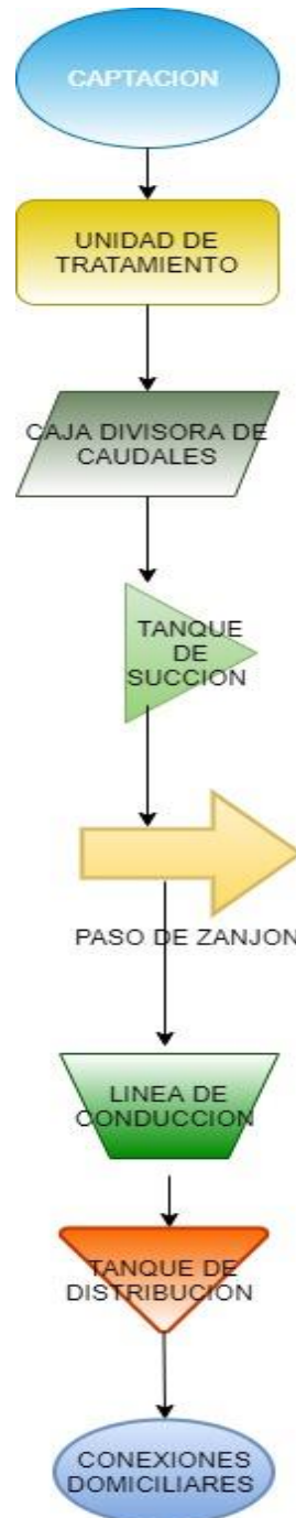
Ilustración 2. Diagrama de flujo del proceso del sistema de agua evaluado.
