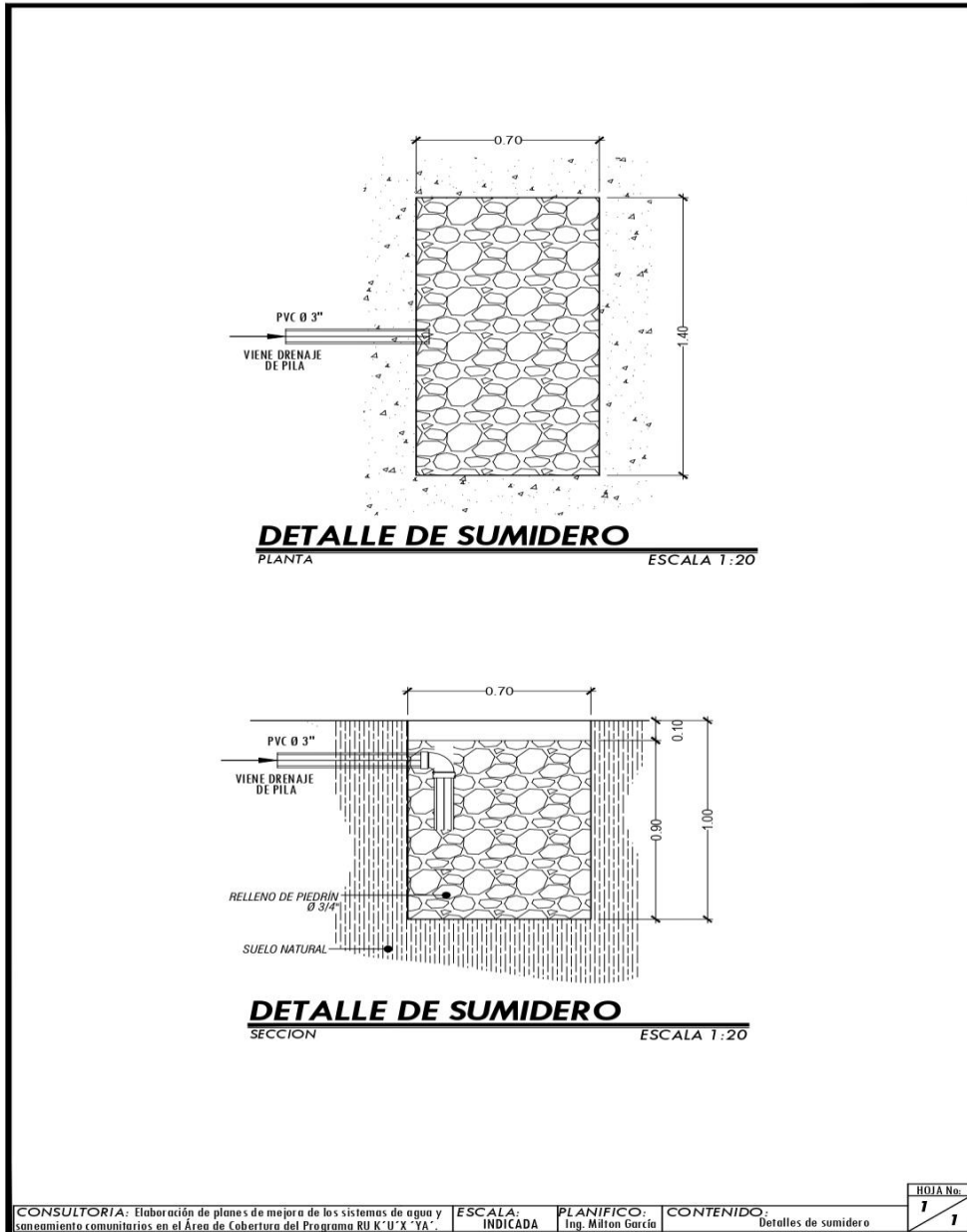
Ilustración 16. Detalle de sumidero.
