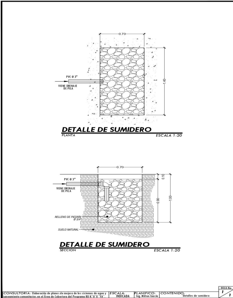
Ilustración 17. Detalle de sumidero.
